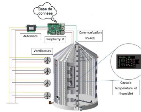
Figure 3 : Idée de conception du procédé automatisé.
